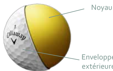
Composition d'une balle 2 pièces
